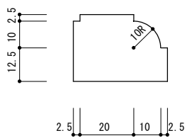
提灯置引き断面図 S=1/2
