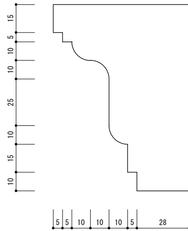
正面置引き断面図 S=1/2
