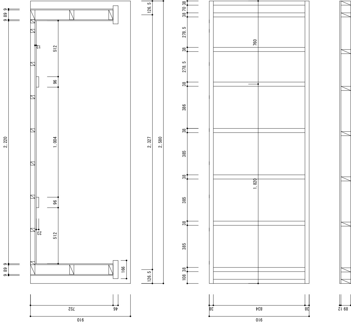
木下地平面図 S=1/20
